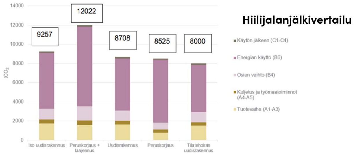
Kuva 20, Tarkasteluvaihtoehtojen elinkaaren hiilijalanjälki jaettuna elinkaarivaiheisiin (tCO 2 )
